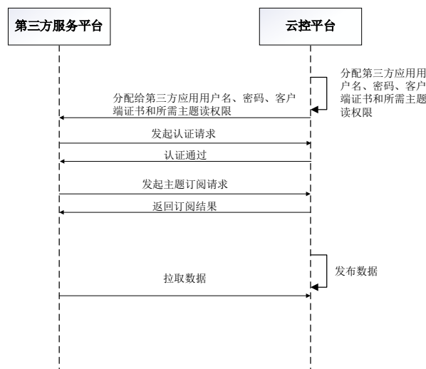
图6 云控平台向第三方服务平台推送数据流程
