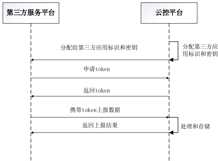
图4 第三方服务平台向云控平台推送数据流程
