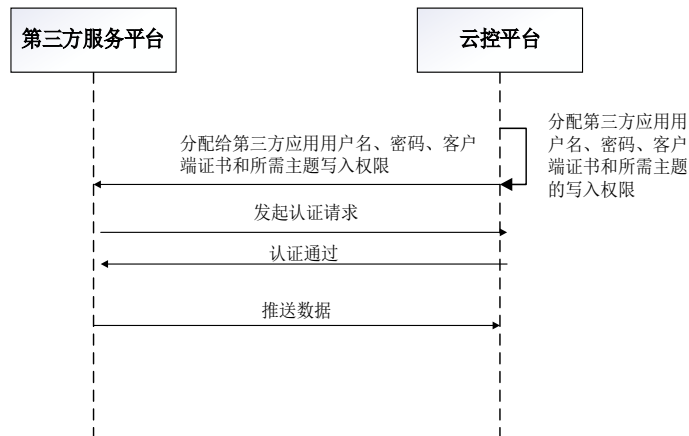
图7 第三方服务平台向云控平台推送数据流程
