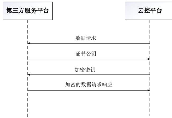
图5 云控平台通过查询方式获取数据流程
