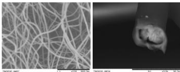
由扫描电子显微镜观测的双 梳理复合面层热风非织造布
